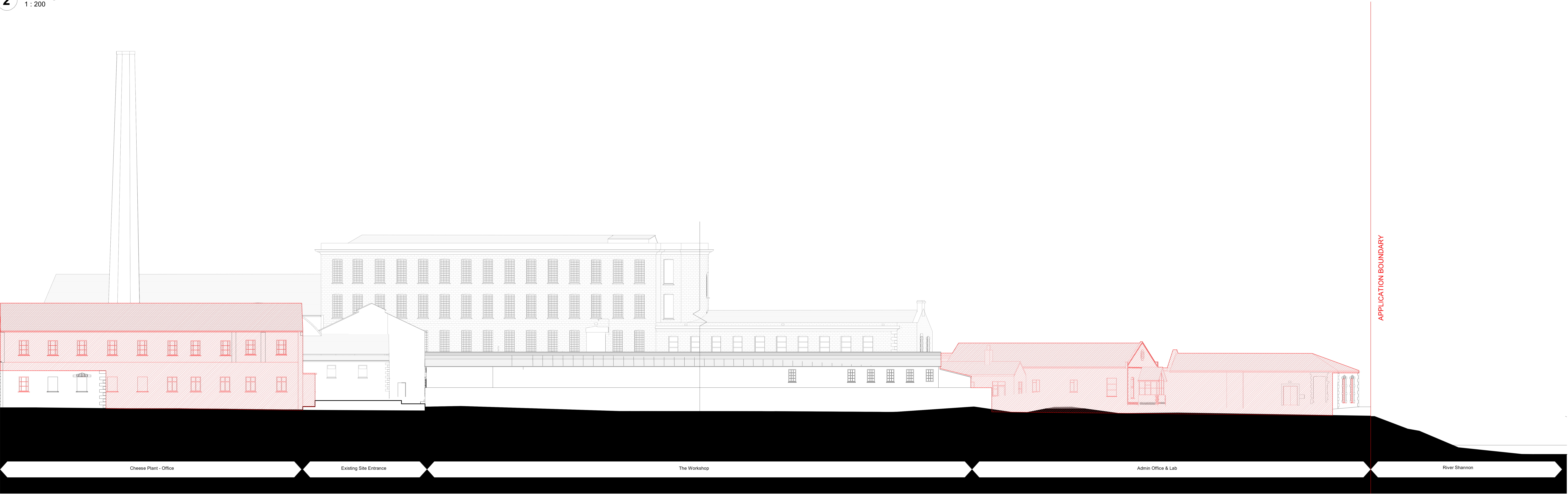
3 Existing Site Elevation - B2 1 : 200
